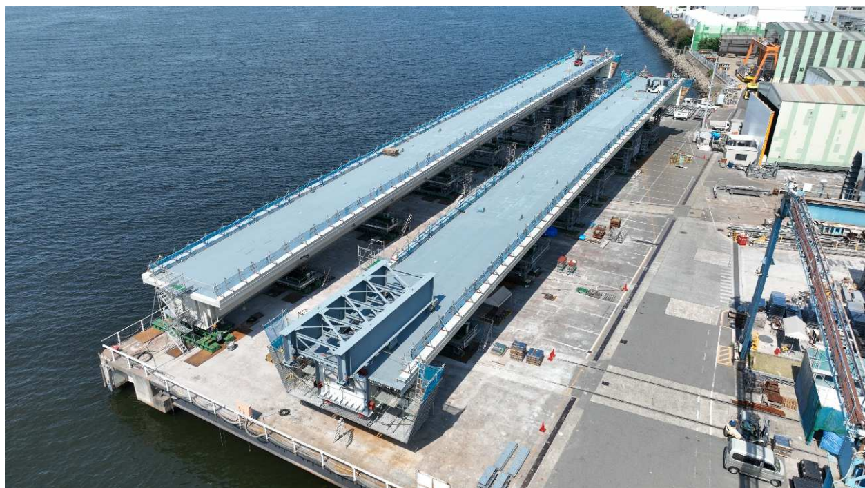
橋桁製作状況（2024.6.14）
