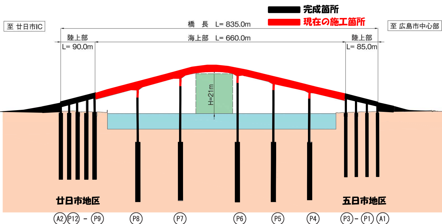
橋桁製作状況（2024.6.14）
