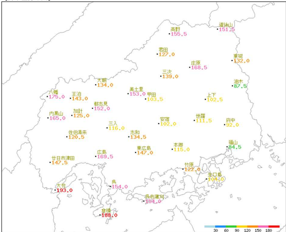
アメダス地点の降水量分布図（令和5年6月29日～7月1日）単位 ミリ
