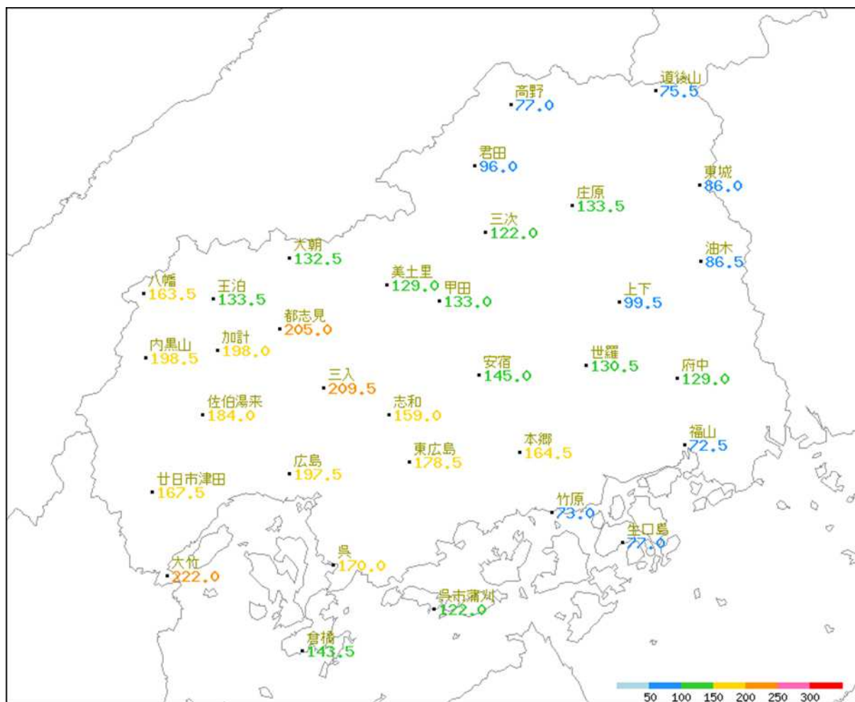
アメダス地点の降水量分布図（令和5年7月7日～7月10日）単位 ミリ
