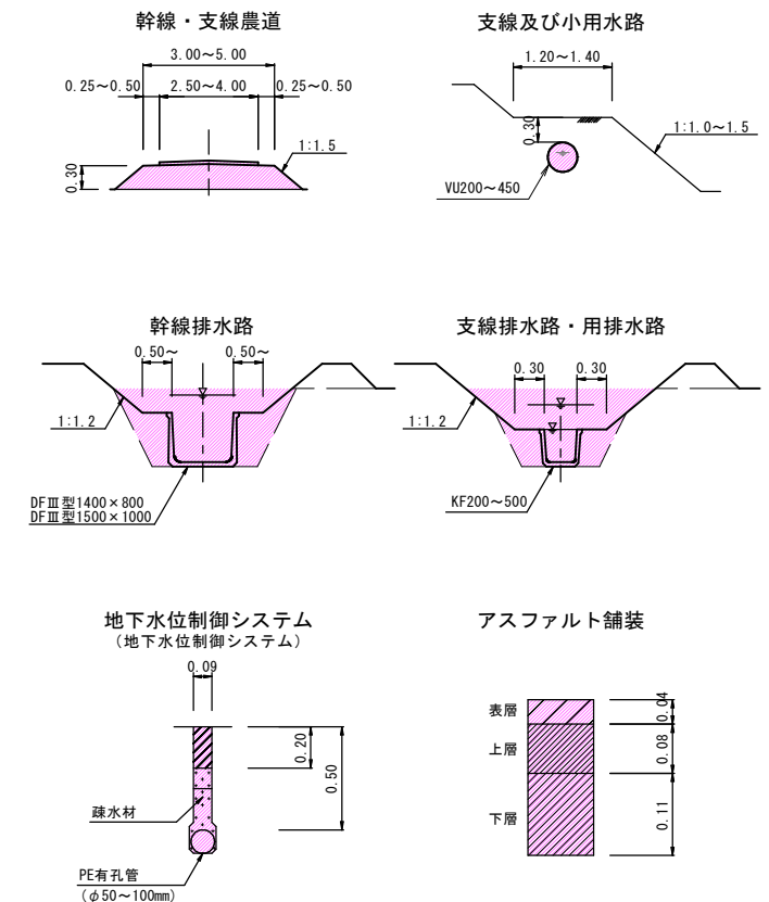
標準断面図
