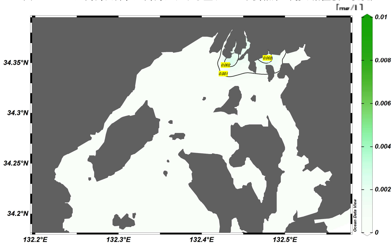
図 3-10-1 広島湾西部、広島湾における全りんの予測結果（増加措置後－現況）
