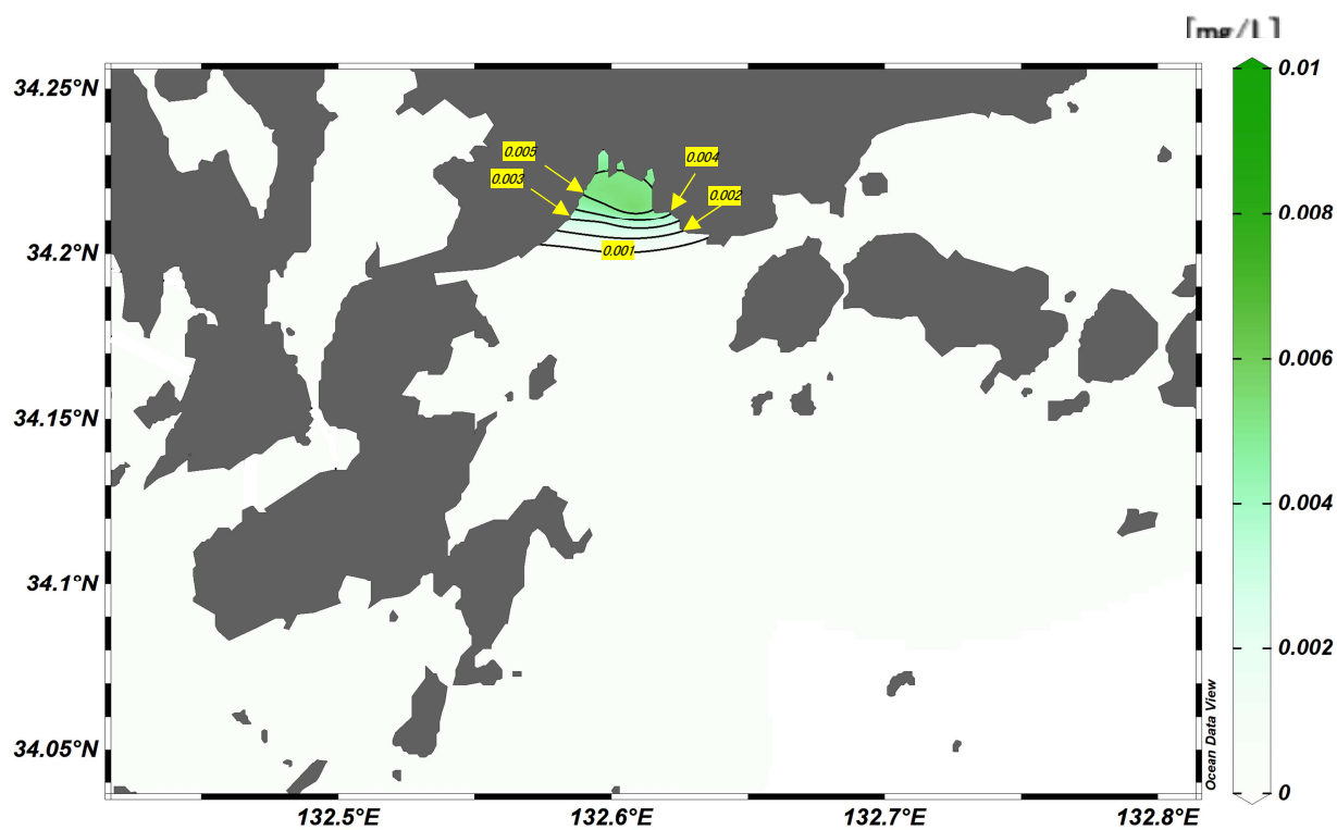
図表 3-10-2 呉地先海域における全りんの予測結果（増加措置後－現況）
