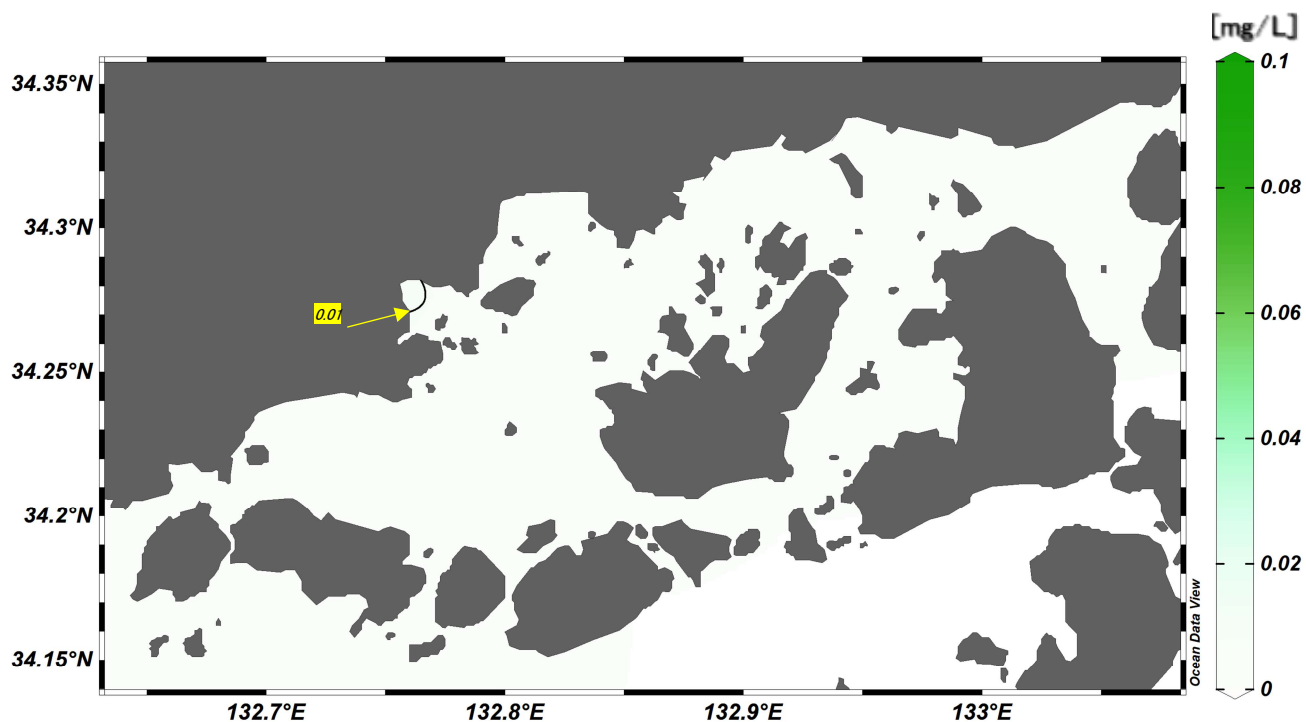
図表 3-9-3 安芸津・安浦地先、燧灘北西部における全窒素の予測結果 (増加措置後－現況)
