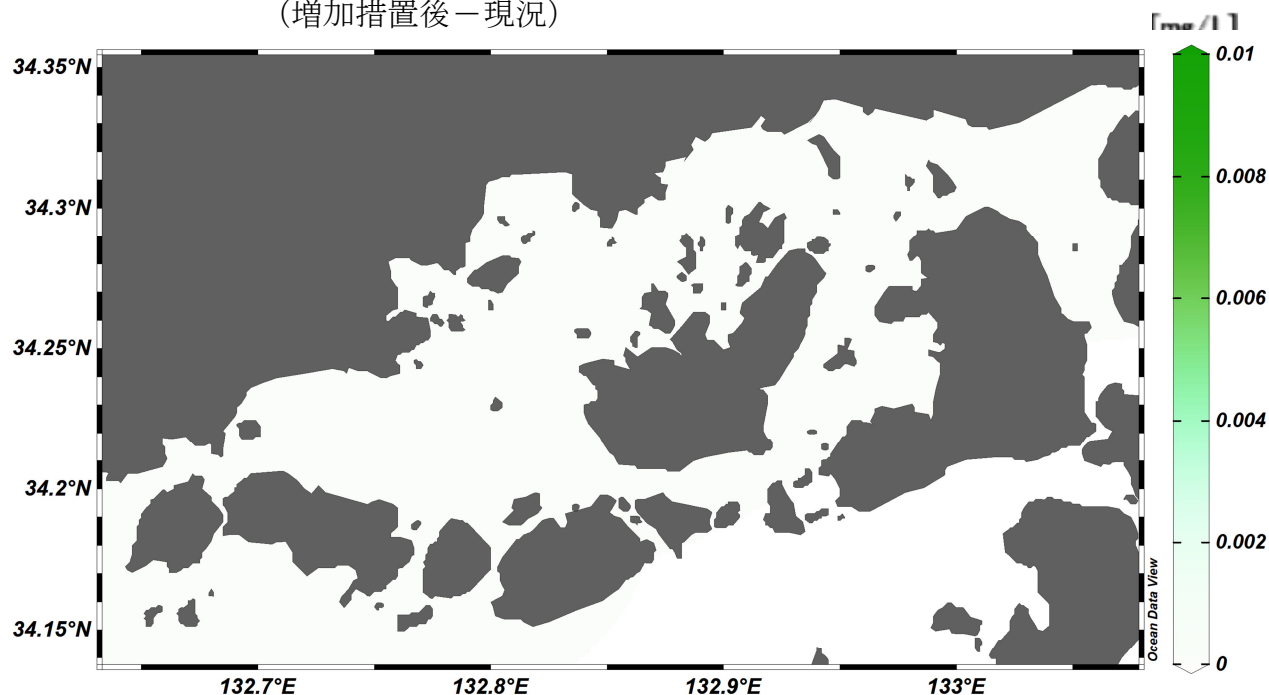
図表 3-10-3 安芸津・安浦地先、燧灘北西部における全りんの予測結果 (増加措置後－現況)
