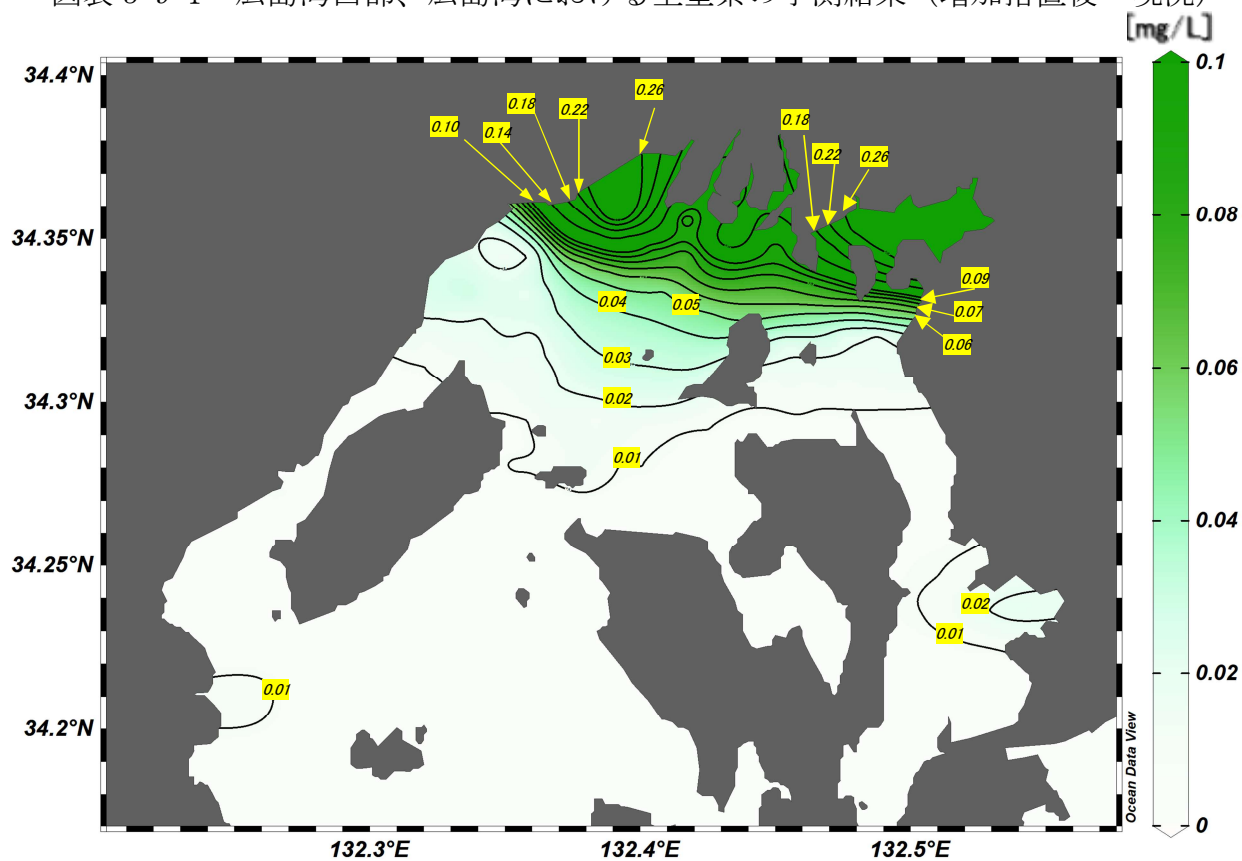
図表 3-9-1 広島湾西部、広島湾における全窒素の予測結果 (増加措置後－現況)
