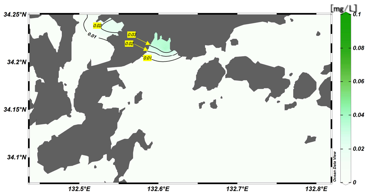
図表 3-9-2 呉地先海域における全窒素の予測結果 (増加措置後－現況)
