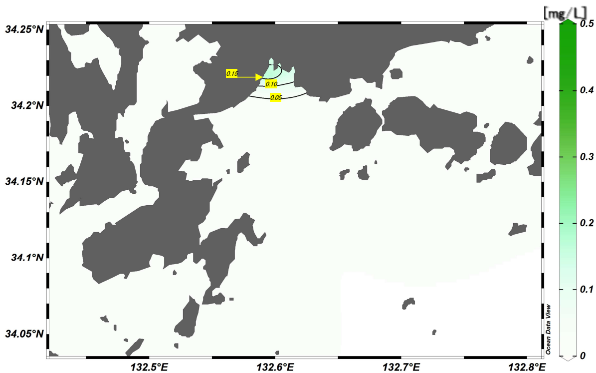
図表 3-11-2 呉地先海域における COD の予測結果 (増加措置後一現況)
