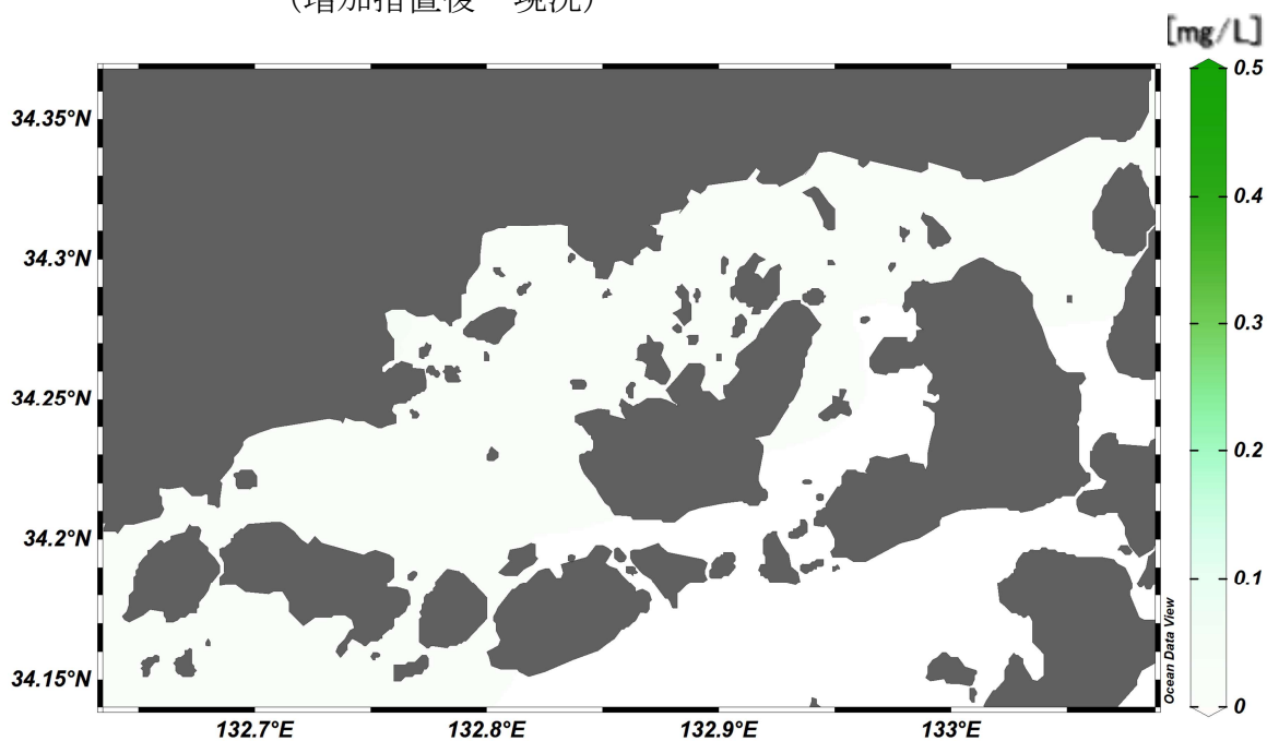
図表 3-11-3 安芸津・安浦地先、燧灘北西部における COD の予測結果 (増加措置後－現況)
