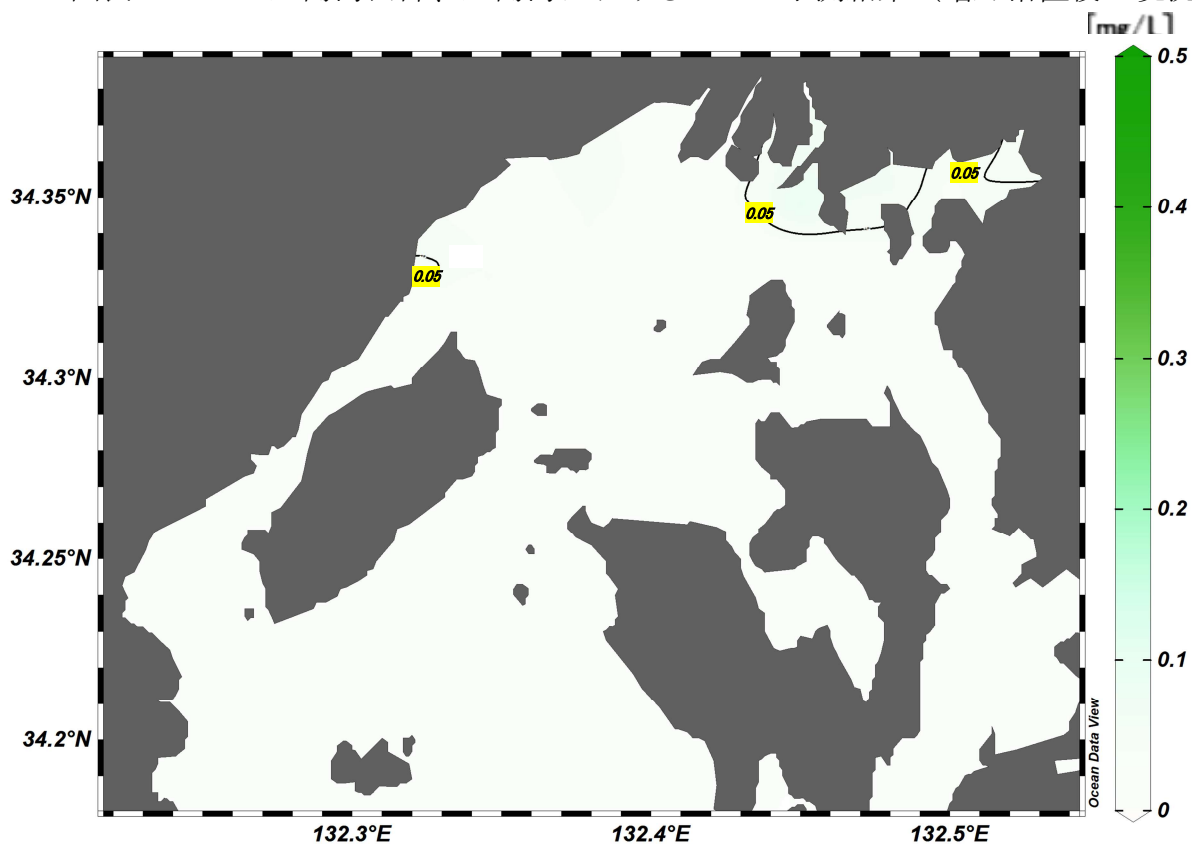
図表 3-11-1 広島湾西部、広島湾における COD の予測結果 (増加措置後一現況)
