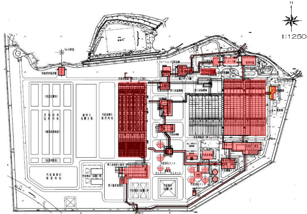
東部浄化センター平面図
