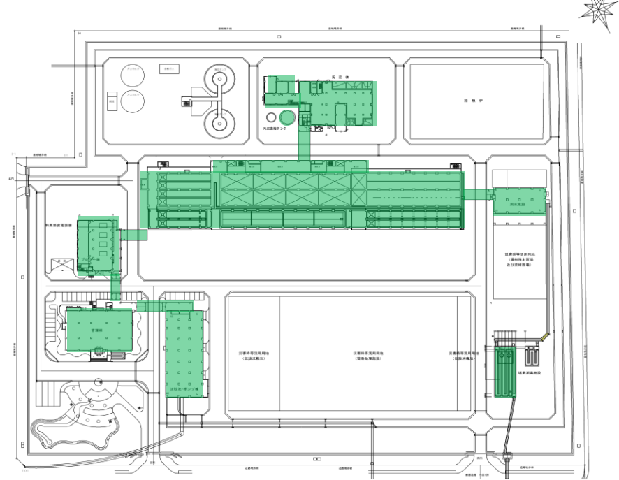
沼田川浄化センター平面図
