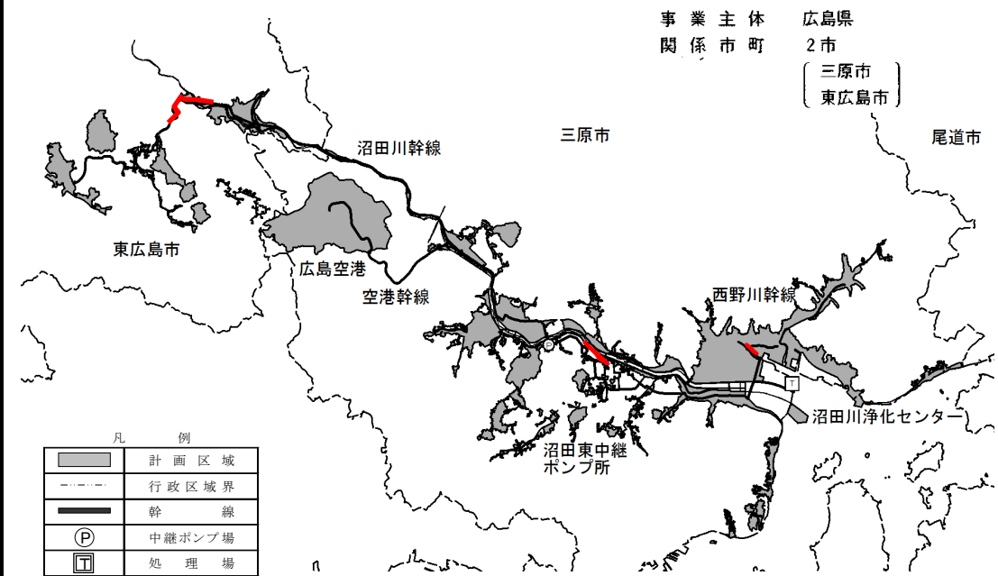
沼田川流域下水道概要図
