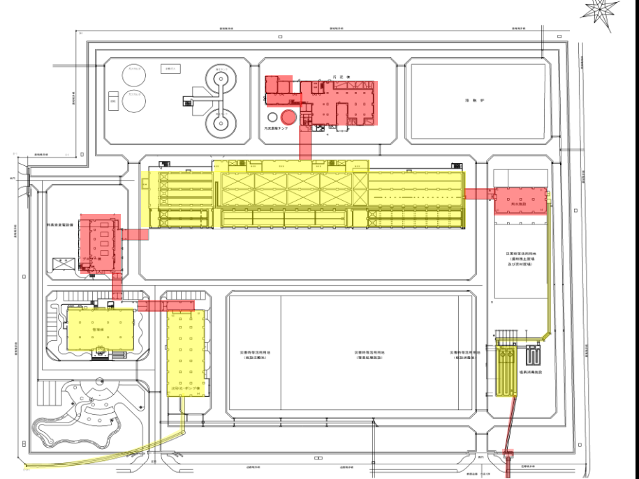
沼田川浄化センター平面図
