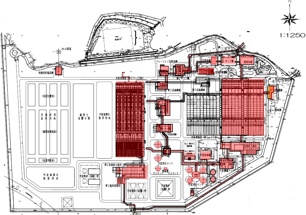
太田川浄化センター平面図
