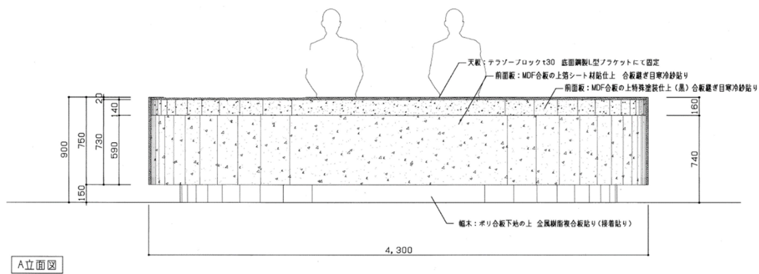
意匠図 (受付台)
