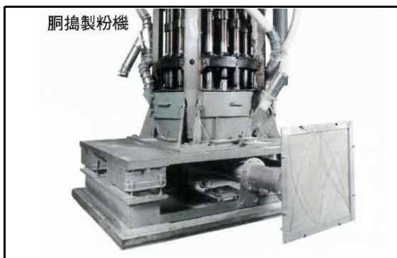
胴搗粉碎機
