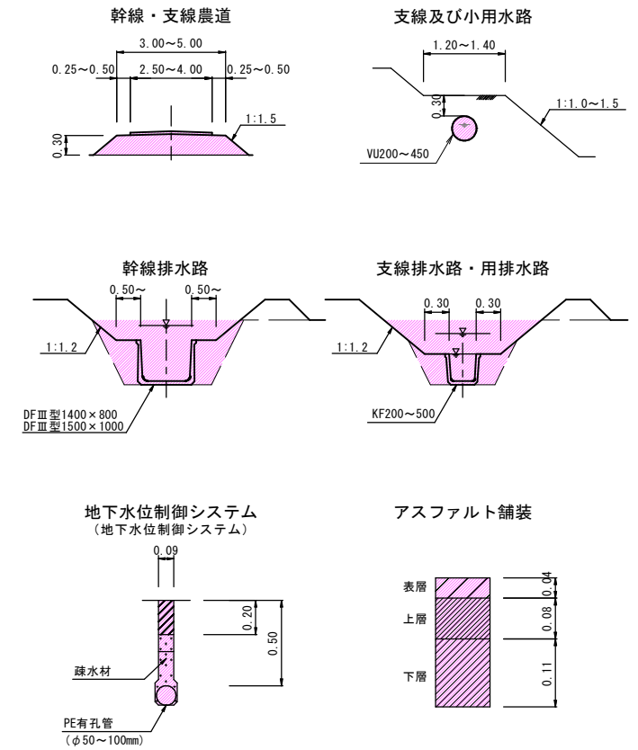
標準断面図
