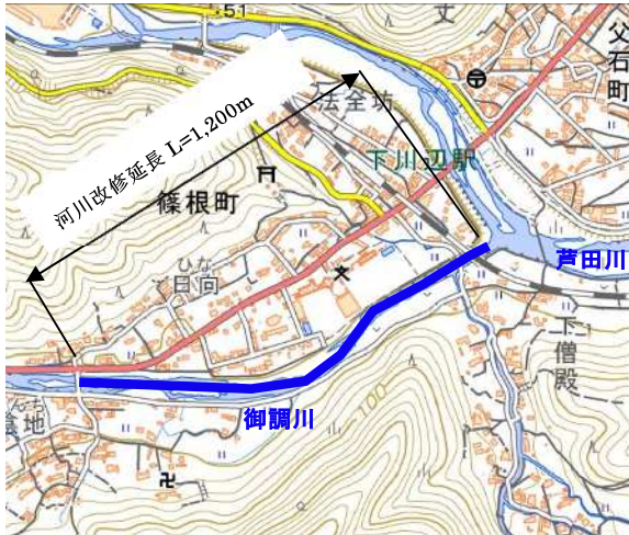
御調川改修計画位置図
