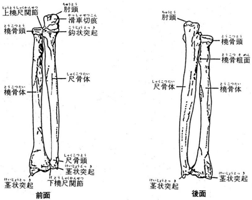
前 腕 骨 (右)
