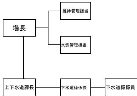
管理体制図
