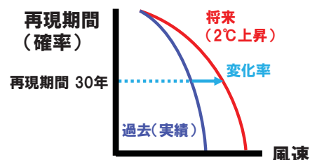
図 気候変動による海上風速の変化率
