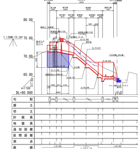
洪水吐縦断面図 H=1/500, V=1/200
