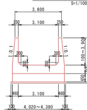
放水路標準断面図
