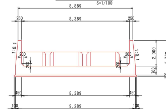
斜樋標準断面図
