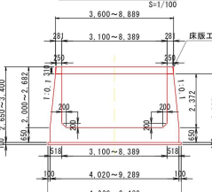
緩勾配水路標準断面図
