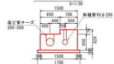
斜樋標準断面図
