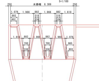
ラビリンス壱平面図
