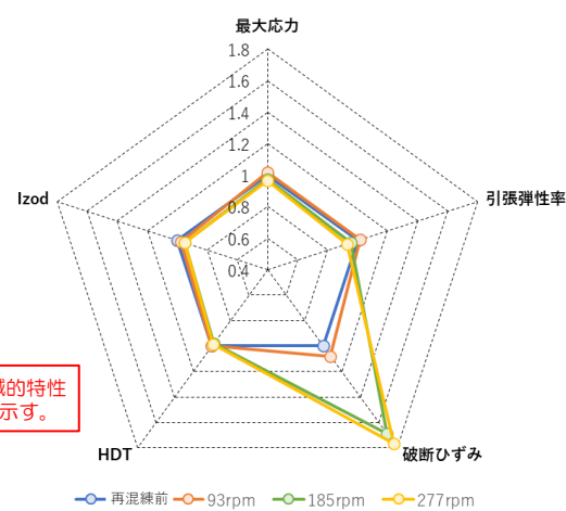
リサイクルペレットでのスクリュ回転数と各種物性の関係※
