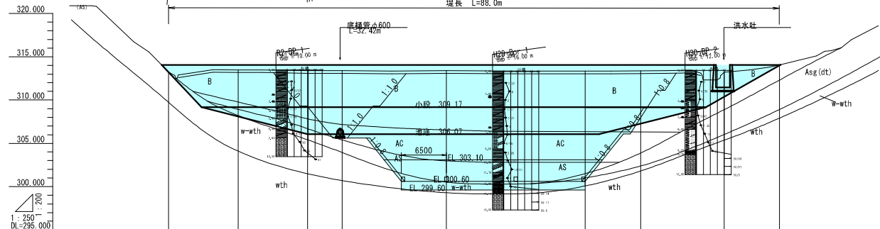
計画縦断面図
