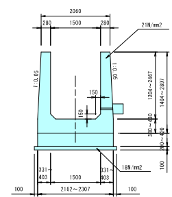
放水路標準断面図
