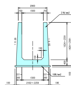
取水施設構造物標準断面図 S=1/5
