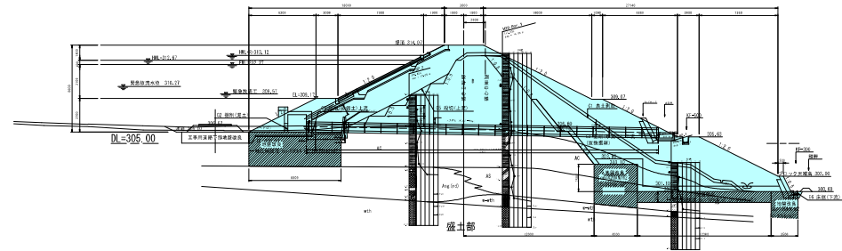
側水路標準断面図
