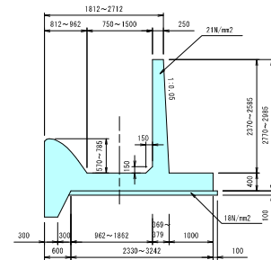
放水路標準断面図
