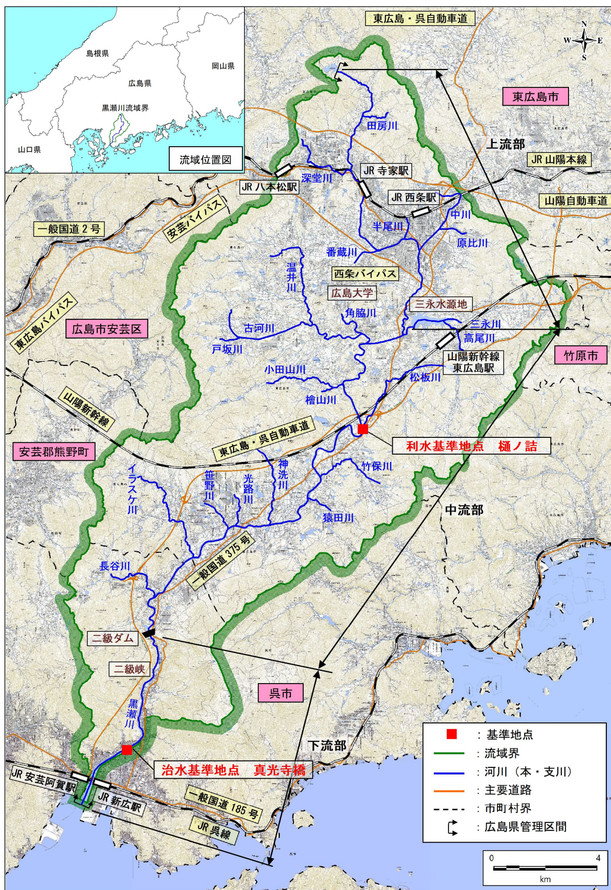
図 黒瀬川水系流域図
