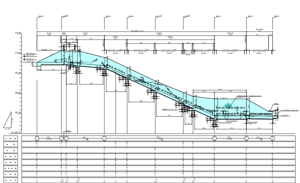
洪水吐工概断面図 S=1/200
