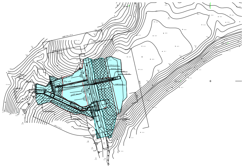
計画平面図 S=1/1000
