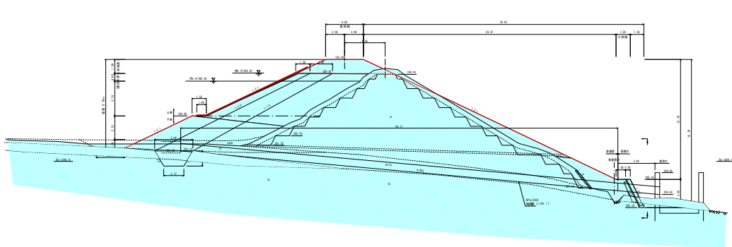
標準断面図 S=1/200
