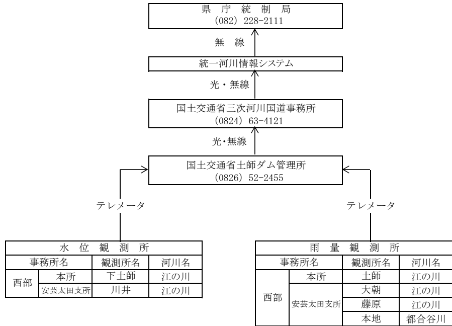
土師ダム系国土交通省水文情報傍受系統図
