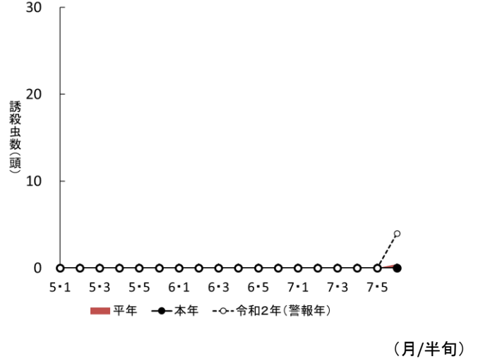
トビイロウンカ 予察灯への誘殺数(八本松町)
