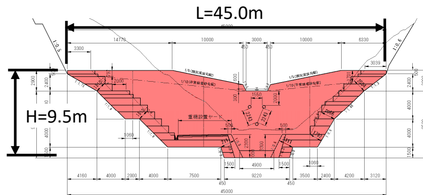
堰堤一般図
