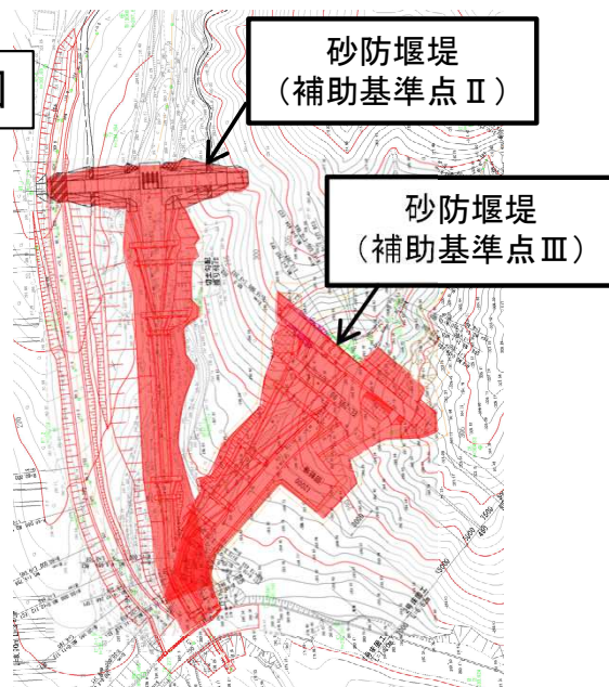
堰堤一般図
