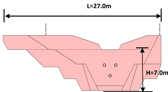
堰堤一般図
