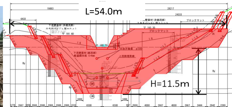
堰堤一般図
