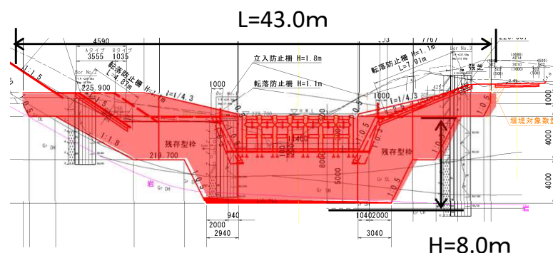
堰堤一般図
