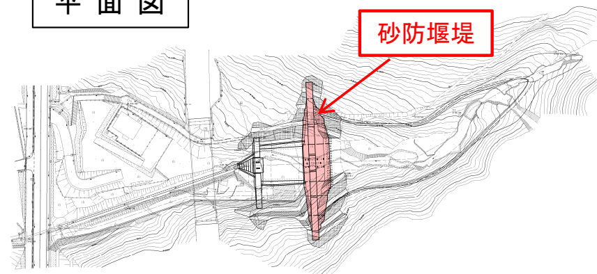
平面図
