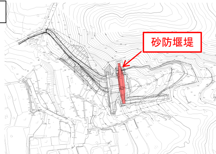
平面図
