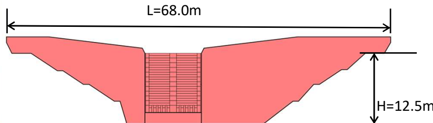
堰堤一般図
