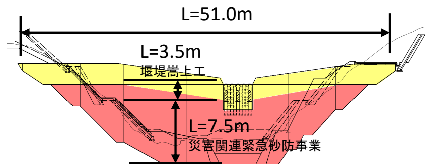
堰堤一般図
