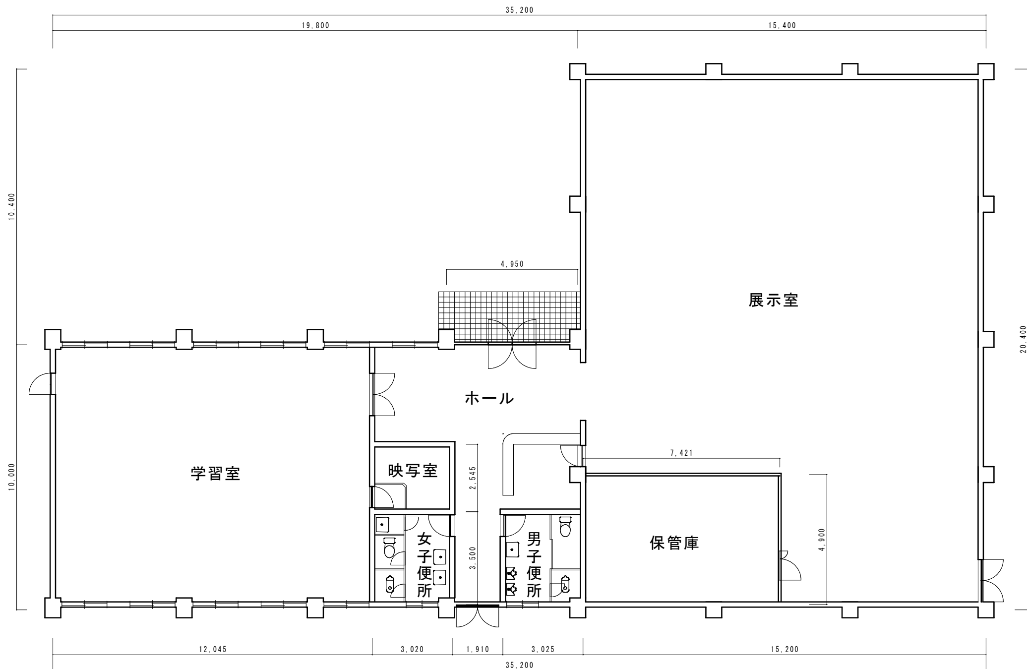
広島県緑化センター 学習展示館 平面図
