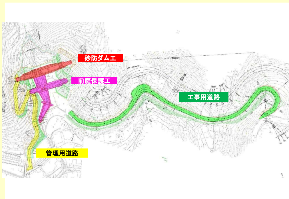
【工事計画平面図】
