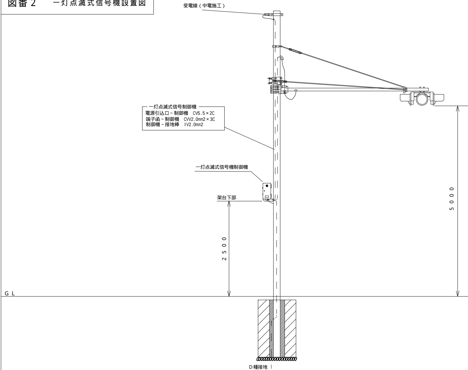
図番 2 一灯点滅式信号機設置図
