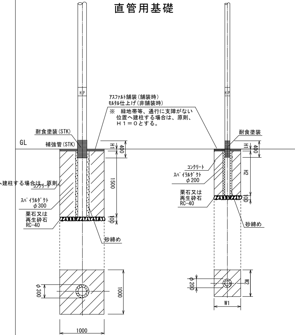
図番 8 専用柱基礎仕様図
