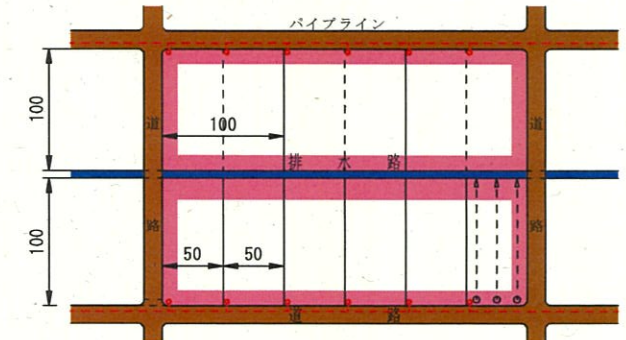
標準断面図
