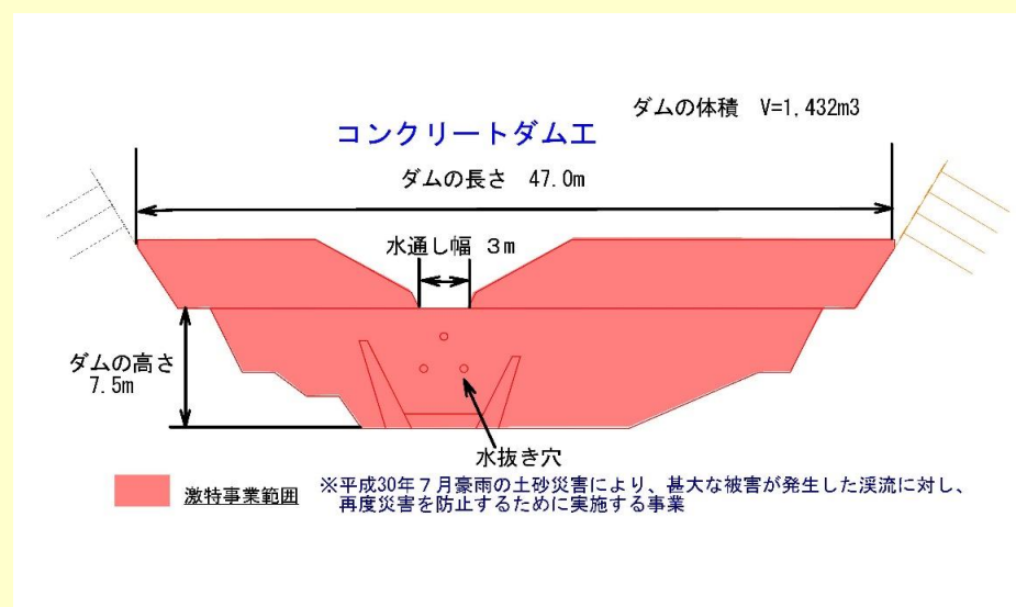
【正面図】
