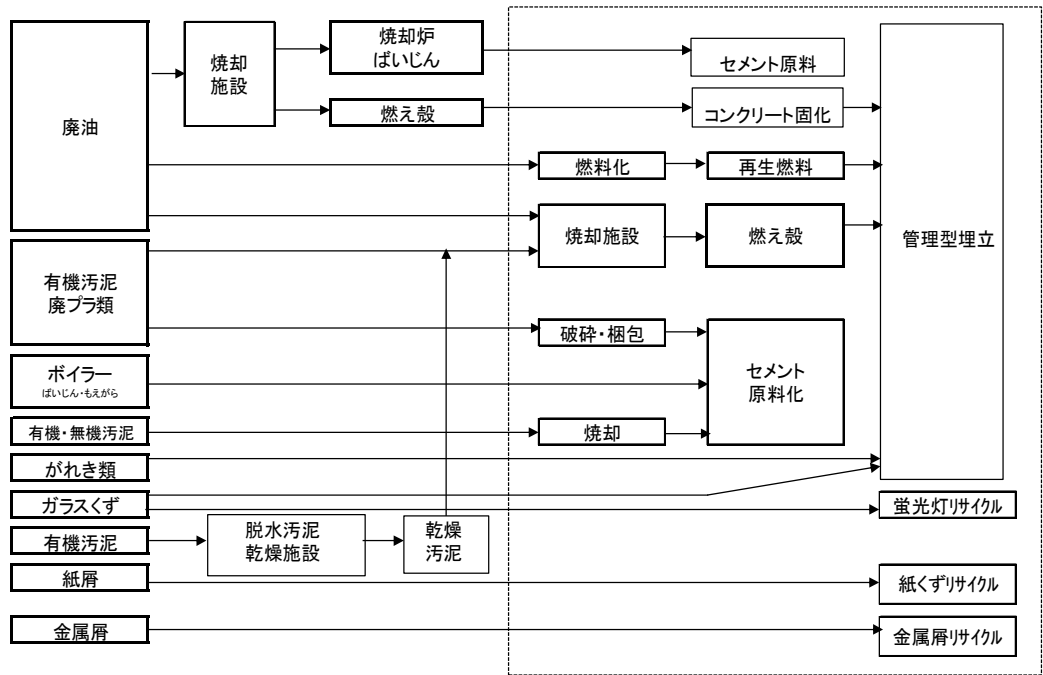
【廃棄物処理フロー図】
