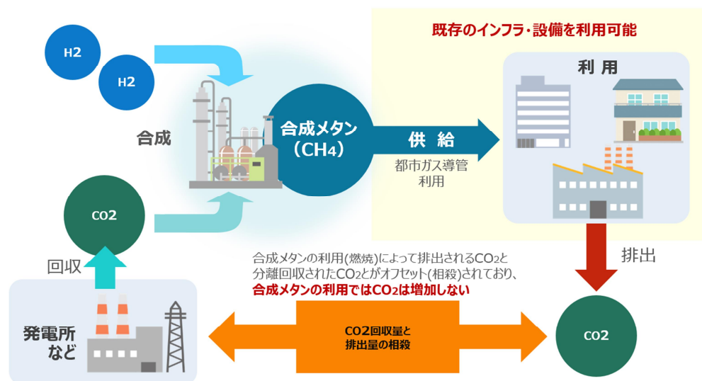
図表 2- 12 メタネーションのイメージ（都市ガス代替燃料利用ケース）
