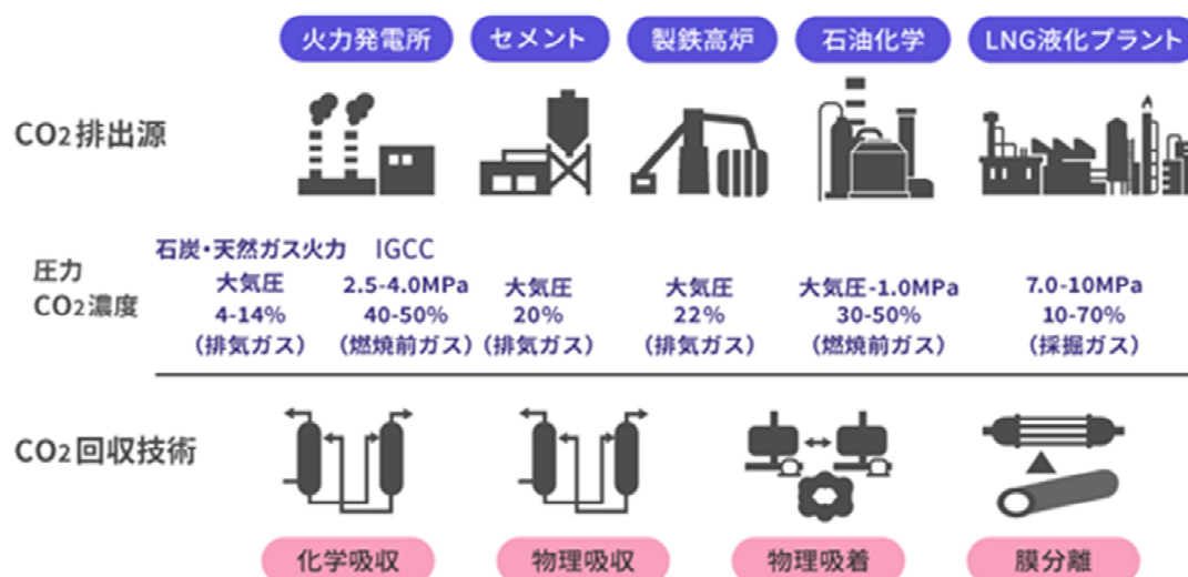
図表2-11 主なCO 2 排出源と分離回収技術
