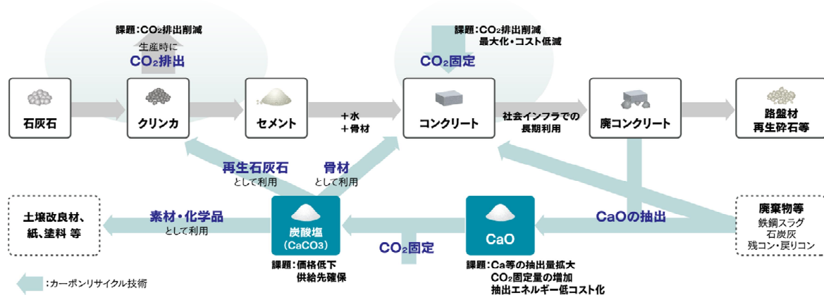
図表 2- 13 カーボンリサイクルコンクリート・セメントの製造イメージ
