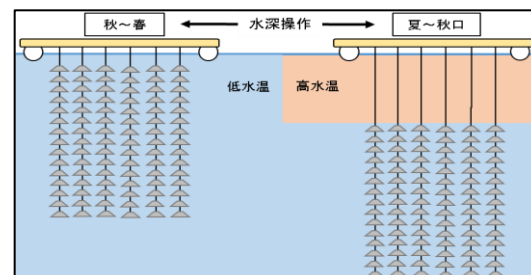
へい死防止対策例
