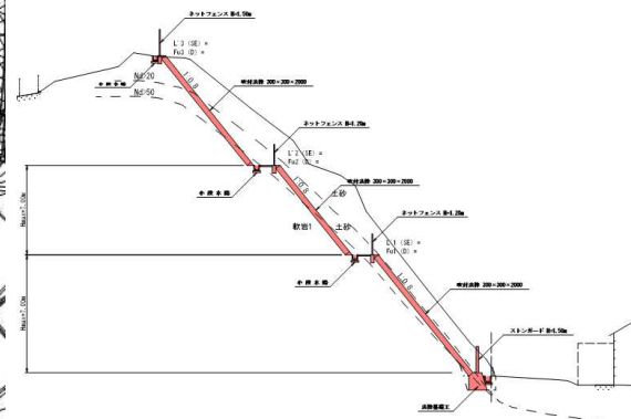
標準断面図
