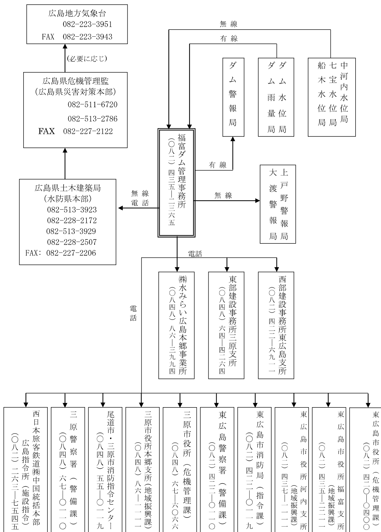
(12) 福富ダム水位雨量等通報系統図
