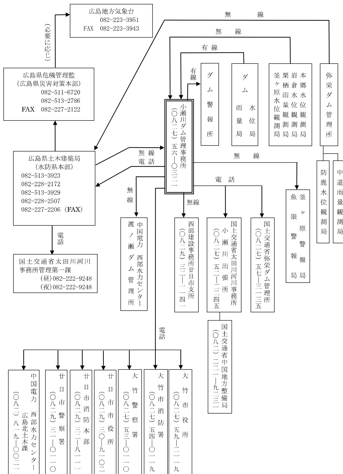
(1) 小瀬川ダム水位雨量等通報系統図
