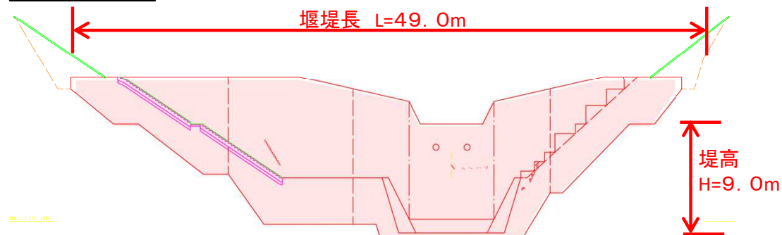
標準断面図
