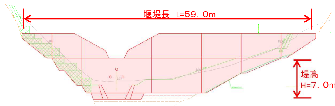
標準断面図
