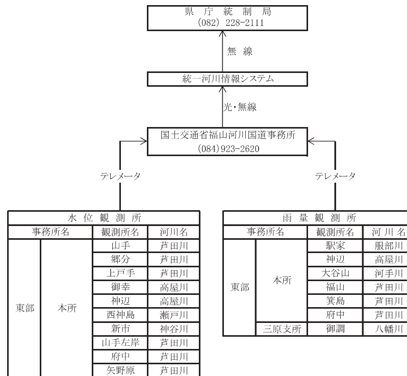
芦田川水系国土交通省水文情報傍受系統図
