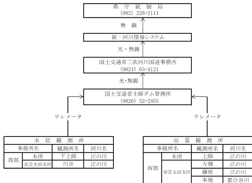
土師ダム系国土交通省水文情報傍受系統図
