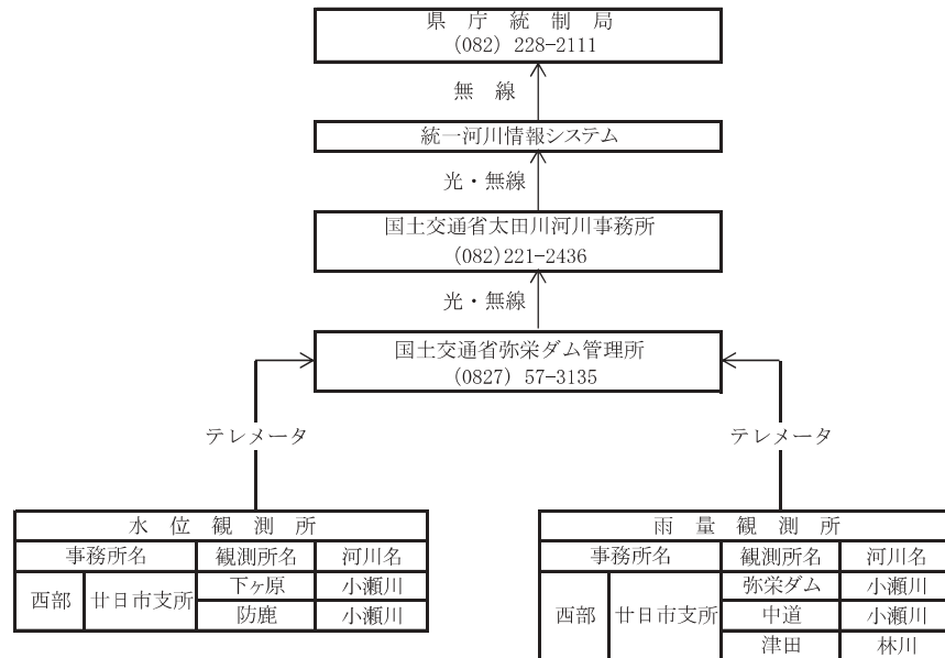
弥栄ダム系国土交通省水文情報傍受系統図
