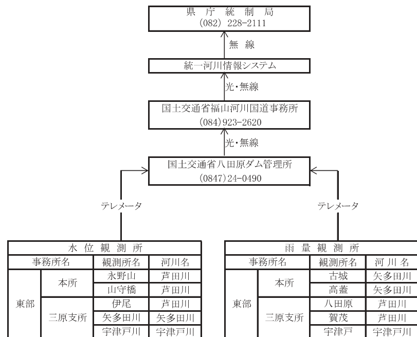
八田原ダム系国土交通省水文情報傍受系統図
