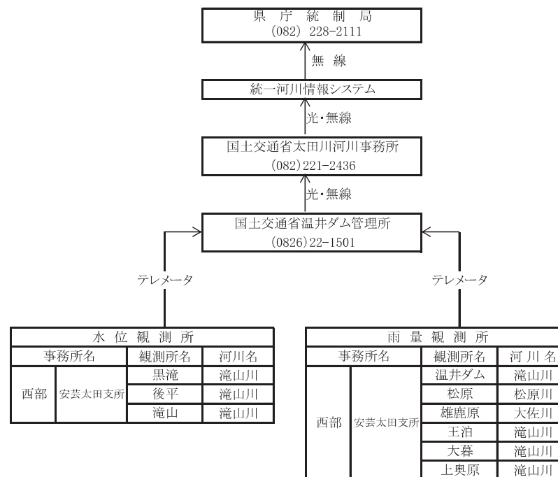
温井ダム系国土交通省水文情報傍受系統図
