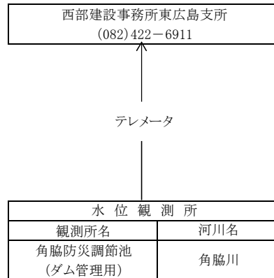
黒瀬川水系広島県水防テレメータ系統図
