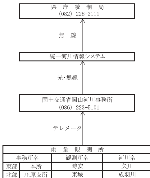
高梁川水系国土交通省水文情報傍受系統図
