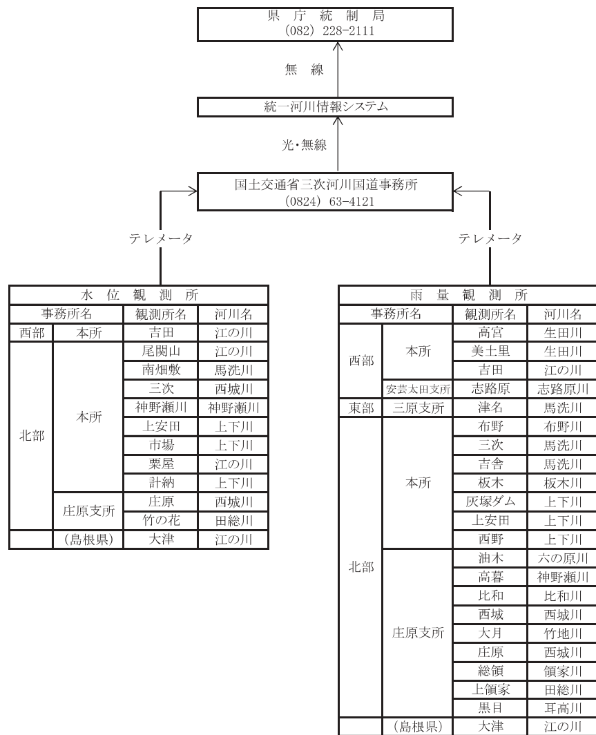
江の川水系国土交通省水文情報傍受系統図
