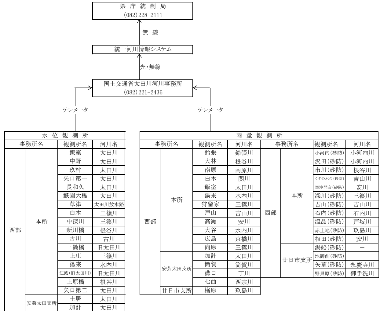
太田川水系国土交通省水文情報傍受系統図
