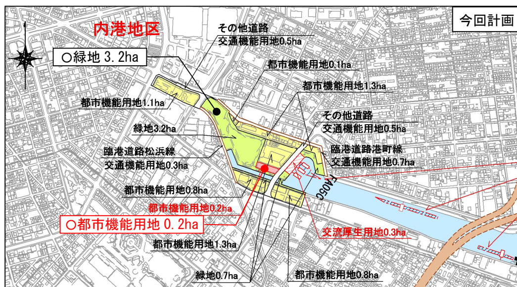
図Ⅲ-1-1 土地利用計画図(内港地区)
