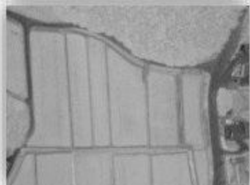
NDVI画像
