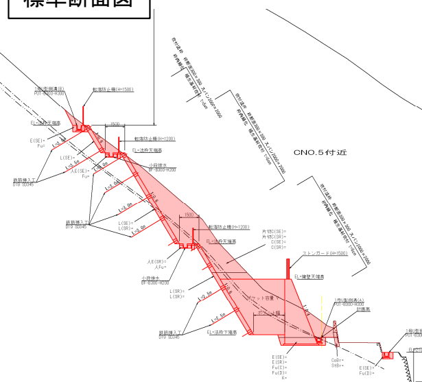
標準断面図
