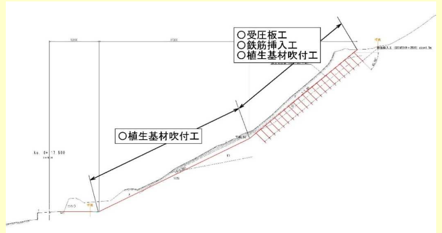
【標準横断図】
