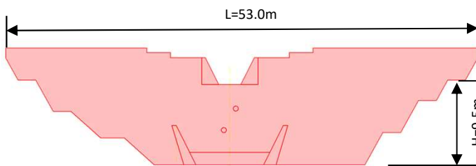
堰堤一般図
