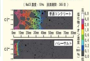
EPMA（電子線マイクロアナライザ）による 表面からの塩化物イオンの浸透深さと濃度解析写真
