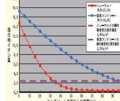
コンクリート表面からの距離と塩化物イオン量の関係 (設計耐用期間：100年、換算塩化物イオン濃度：0.015(%) 2 (伊賀区庁参考値))
