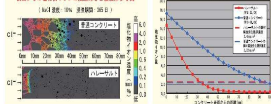
EPMA（電子線マイクロアナライザ）による表面からの塩化物イオンの浸透深さと濃度解析写真
